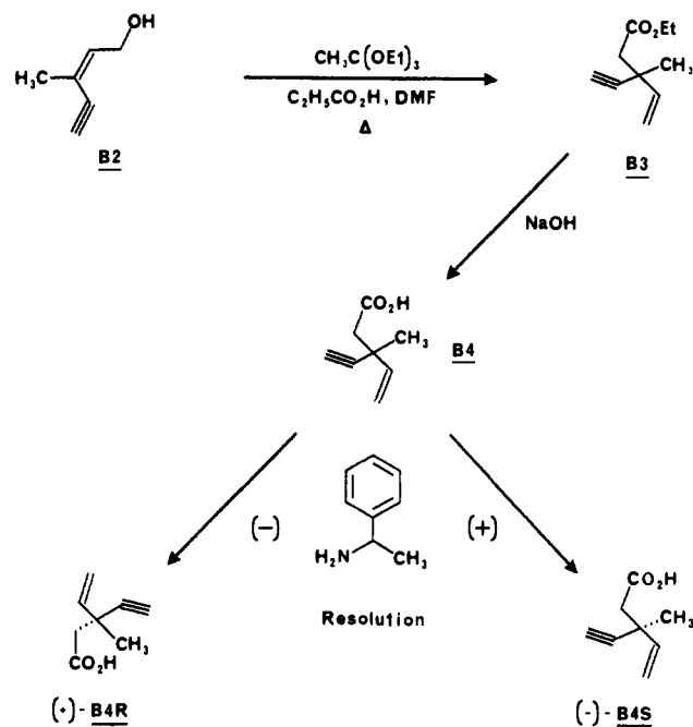
Scheme VI
